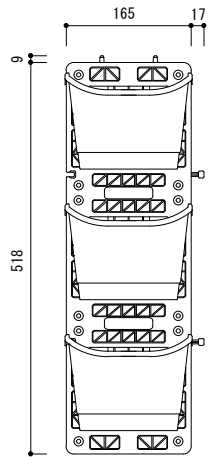
正面図
